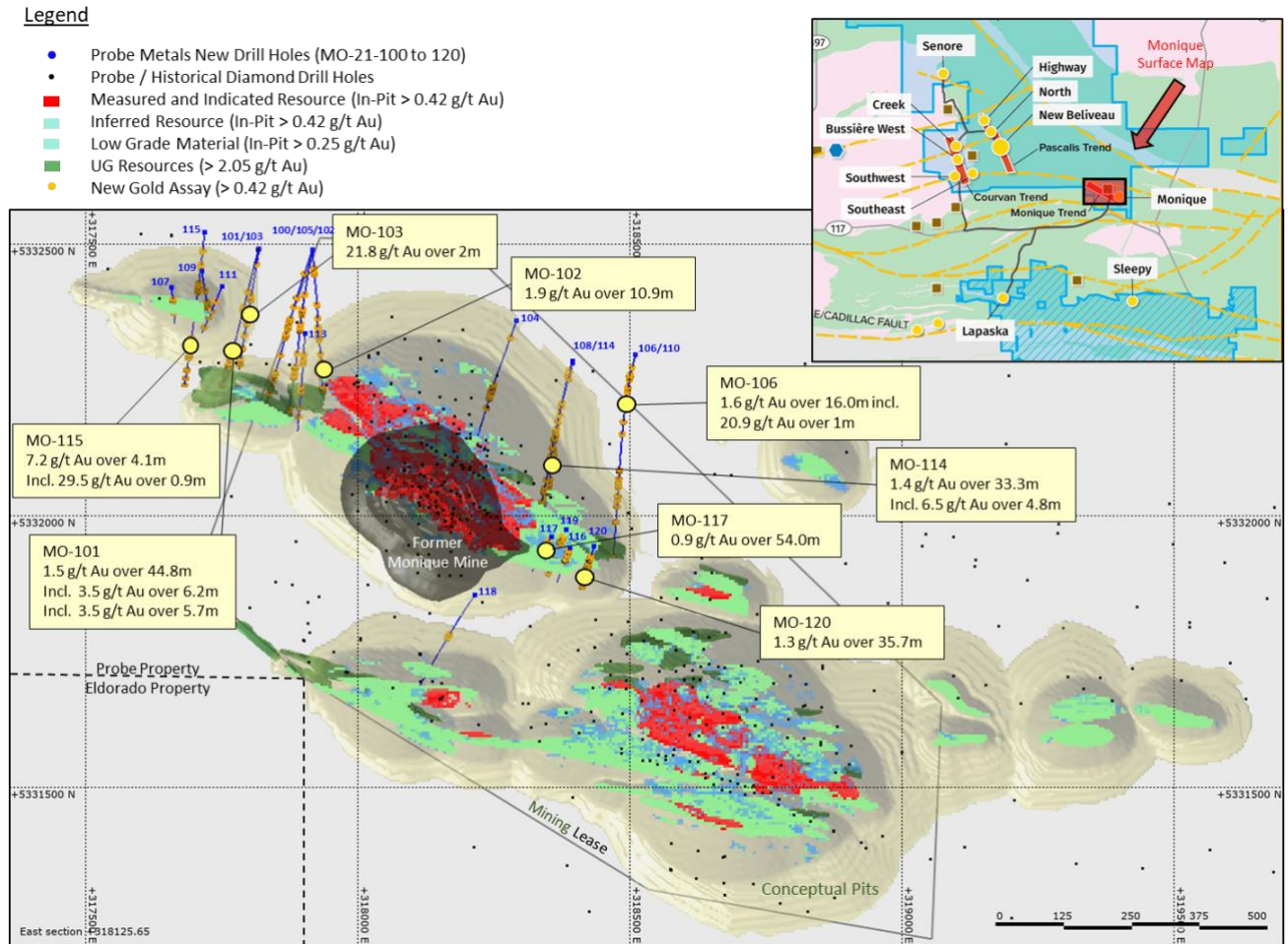
Figure 1 : Plan de surface – Nouveaux résultats de forage le long du couloir aurifère Monique
