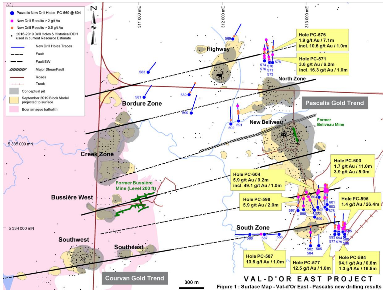
Figure 1 Plan de surface – Val-d'Or Est – couloir aurifère de Pascalis
